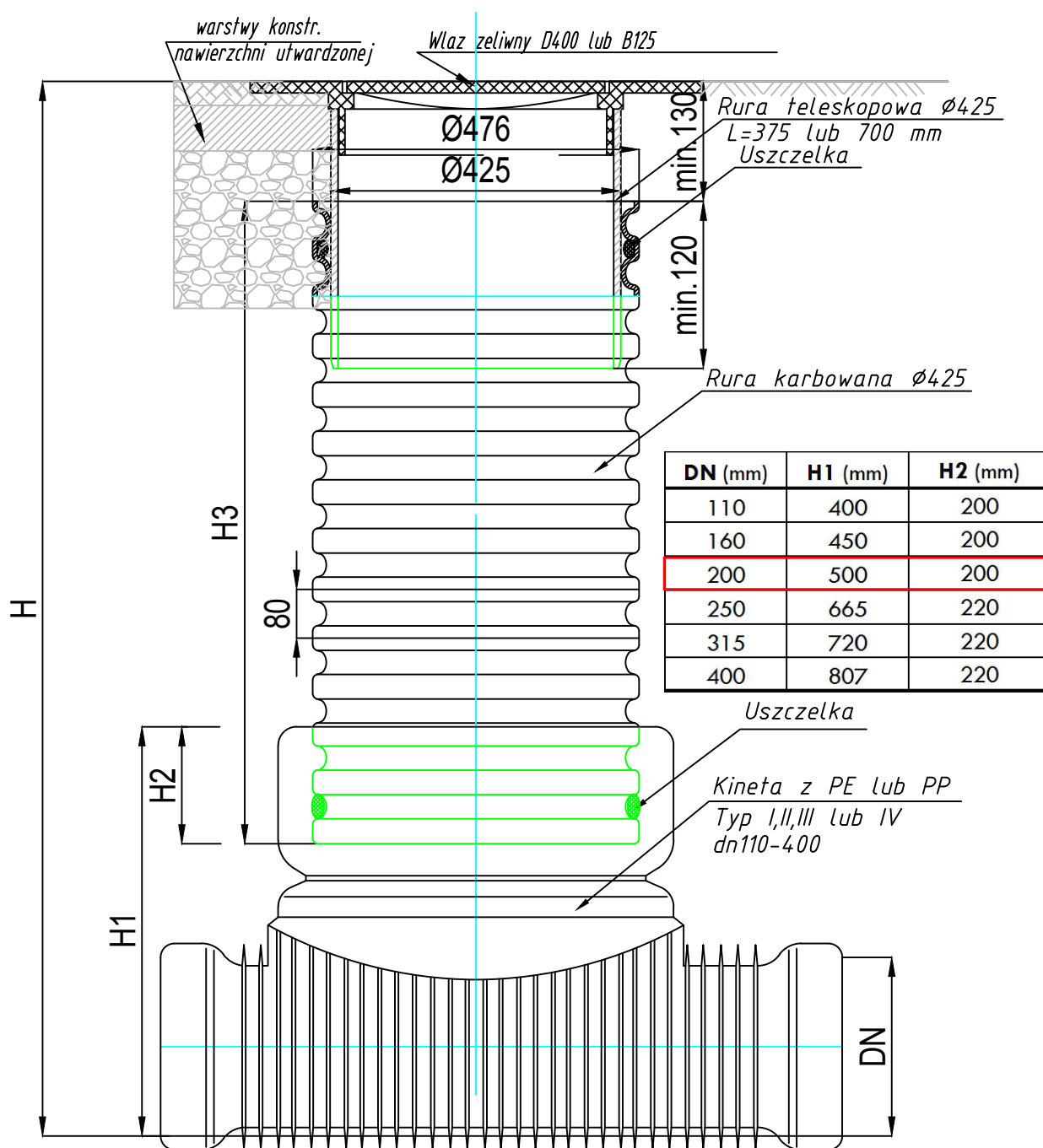
Studzienka inspekcyjna \varnothing 425 z rura teleskopowa i włazem zeliwnym klasy D400 lub B125
