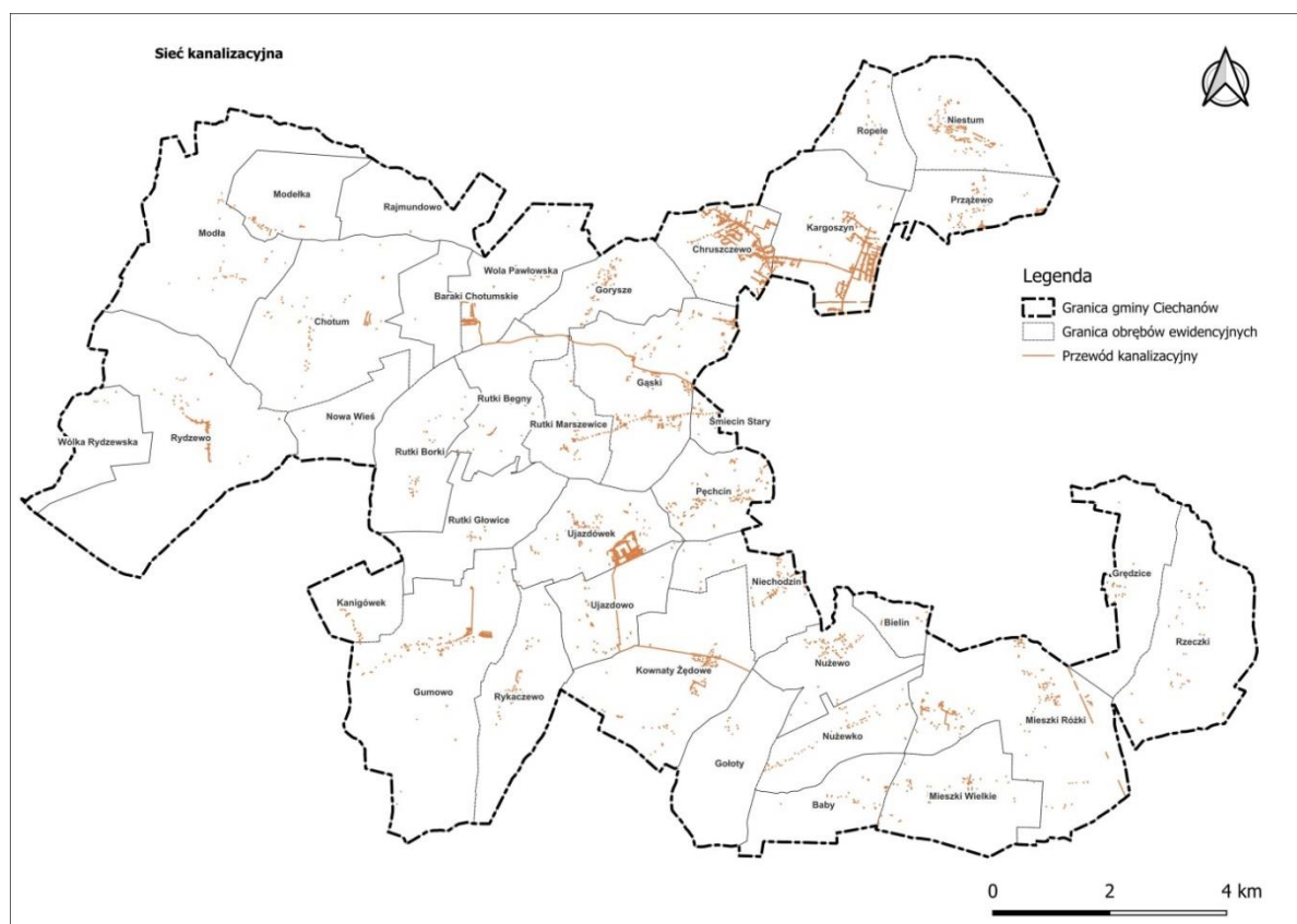
Ryc. 23. Sieć kanalizacji sanitarnej na terenie gminy Ciechanów
