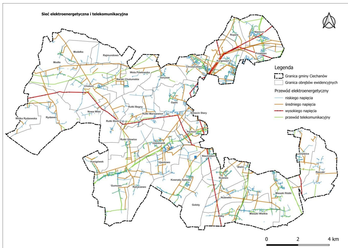
Ryc. 10. Sieć elektroenergetyczna i telekomunikacyjna na terenie gminy Ciechanów
