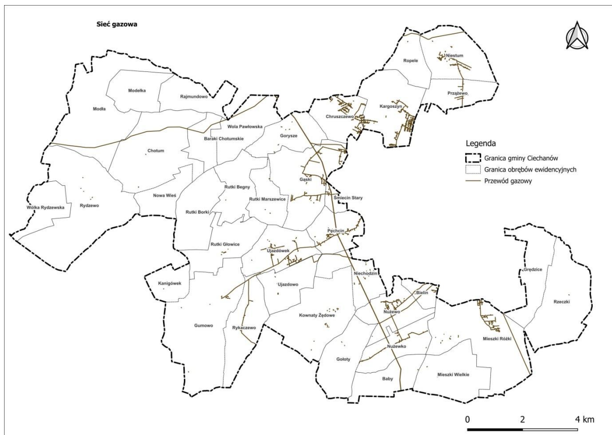
Ryc. 9. Sieć gazowa na terenie gminy Ciechanów
